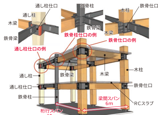
木造・鉄骨共存型ハイブリッド架構のイメージ
