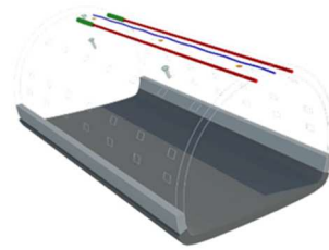
① 通常施工（肩部まで）
