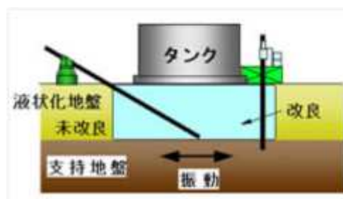
注入固化工法のイメージ図
