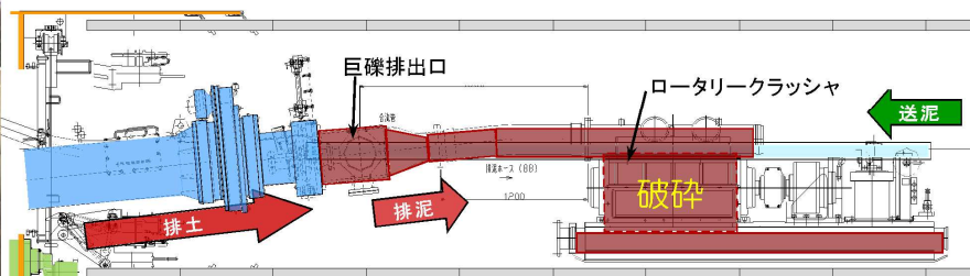
ロータリークラッシャー装備の例
