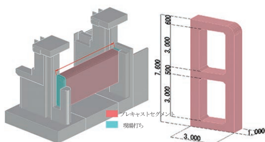
図-1 カーテンウォール正面・断面図
