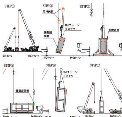
図-2 施工手順概要図
