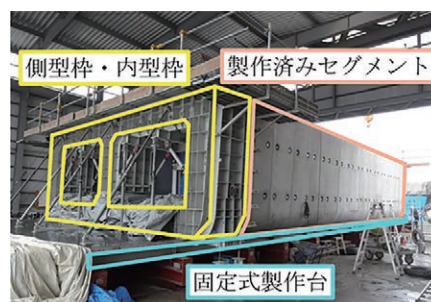
写真-1 セグメント製状況
