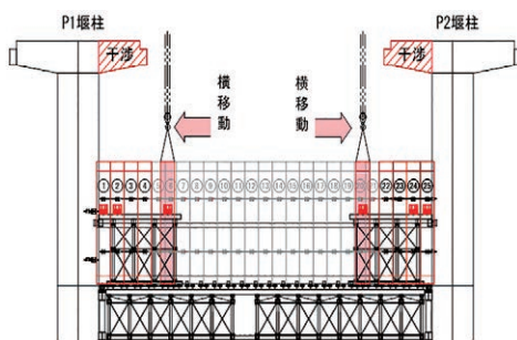
図-3 横移動による架設計画図
